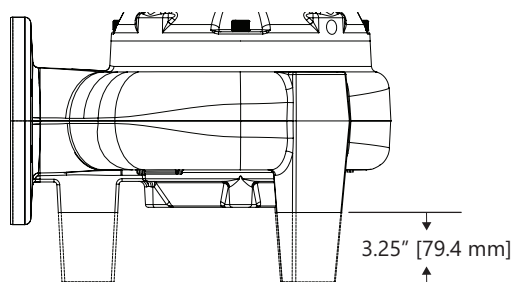
Figura 1. Punto de corte para bombas de 3 a 5 hp
